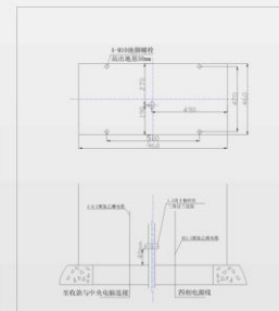
底座安装图
